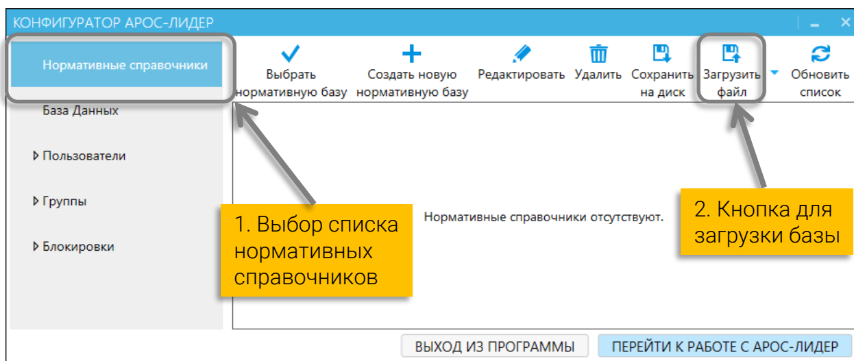
Рис.2. Окно конфигуратора «АРОС-Лидер 2.0»
