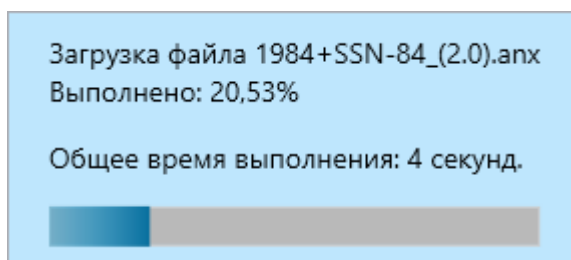
Рис.4. Индикатор выполнения
